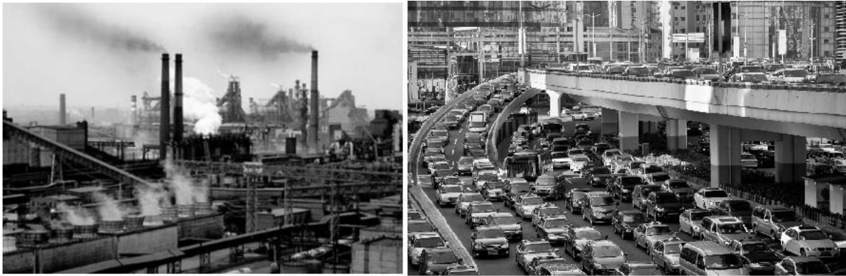
Рис. 6. Загрязнения среды. Техногенные не восстанавливаемые ландшафты
